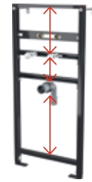
A104A/1120 Montažni ram za umivaonik i bateriju
