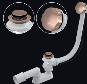
A55K-RG-P Sifon za kadu automatski, RED GOLD-sjaj
