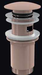
A392-RG-P Gornji deo sifona za umivaonik CLICK/CLACK 5/4" metalni sa prelivom, veliki čep, RED GOLD-sjaj
